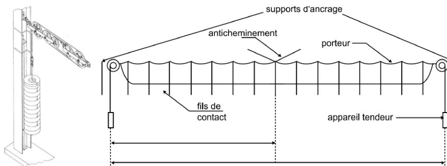
Figure 1.6 – a. (gauche) Appareil tendeur à mouffes ; b. (droite) Canton de pose.
