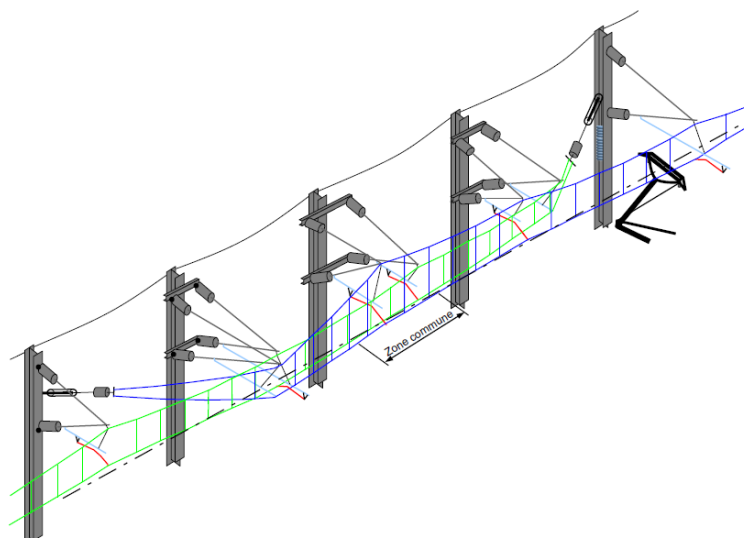
Figure 1.7 – Équipement tendeur de type 25 kV.
