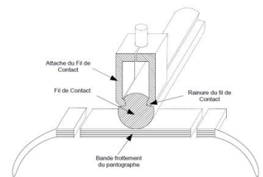
Figure 1.2 – Coupe du fil de contact et du pantographe.
