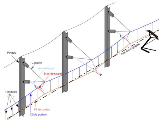
Figure 1.3 – Représentation de la caténaire de type 25 kV sans câble Y.
