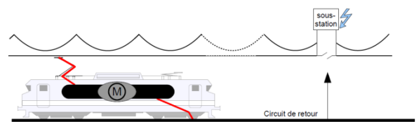
Figure 1.1 – Schéma de circulation du courant électrique.
