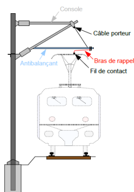
Figure 1.4 – Schéma d'une ligne aérienne de traction électrique.
